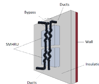
SMHRU Unità modulare di recupero calore
