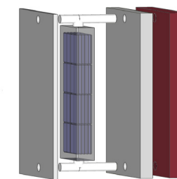
LHTES Sistema di stoccaggio di energia termica latente
